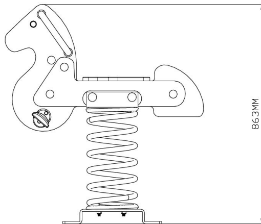
Zijaanzicht
