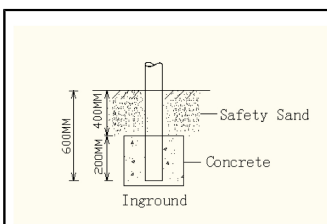
Betonfundatie
