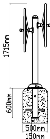
Vooraanzicht
