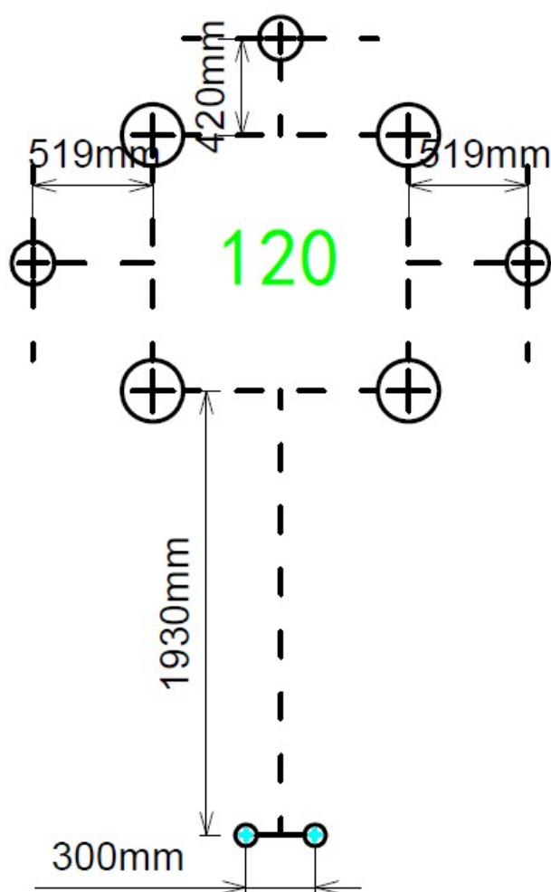
Plattegrond palenplan
