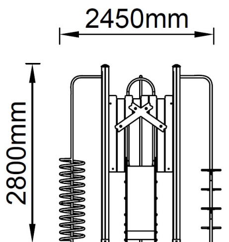
Vooraanzicht
