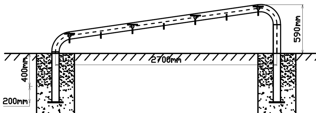
Zijaanzicht
