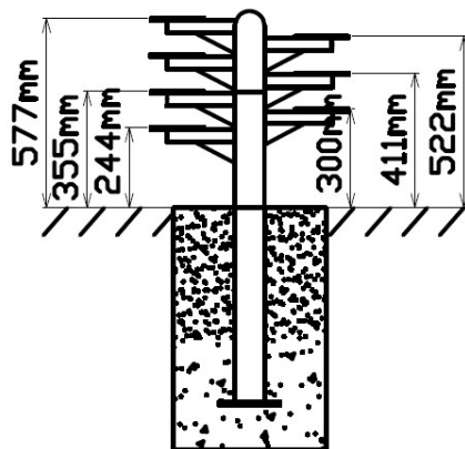
Vooraanzicht
