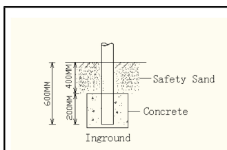
Betonfundatie
