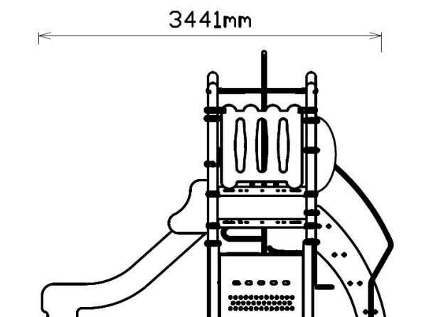
Zijaanzicht
