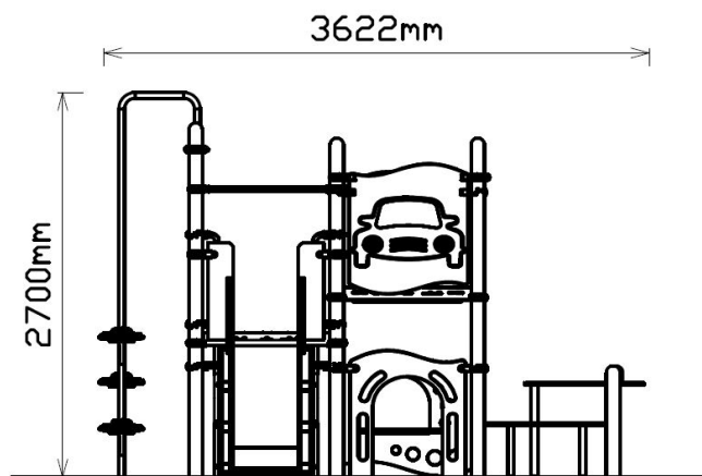
Vooraanzicht
