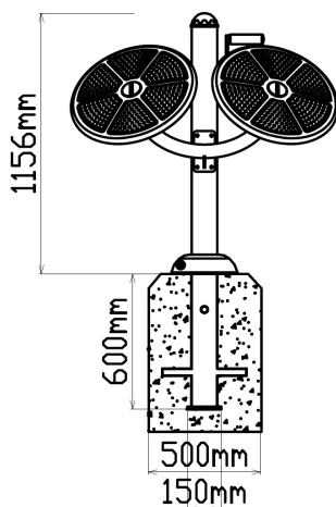
Zijaanzicht
