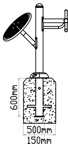
Vooraanzicht
