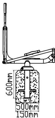
Vooraanzicht
