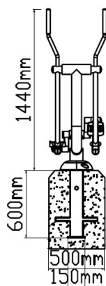
Zijaanzicht
