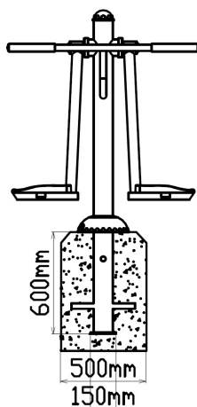
Vooraanzicht
