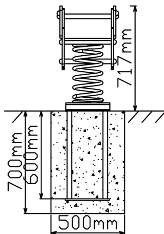
Vooraanzicht
