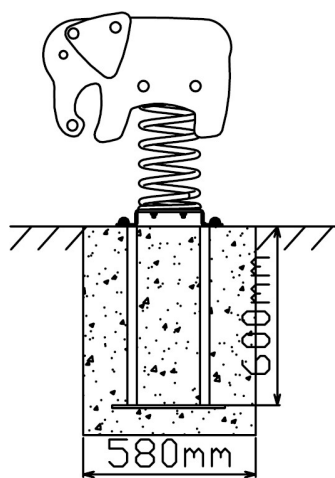
Zijaanzicht
