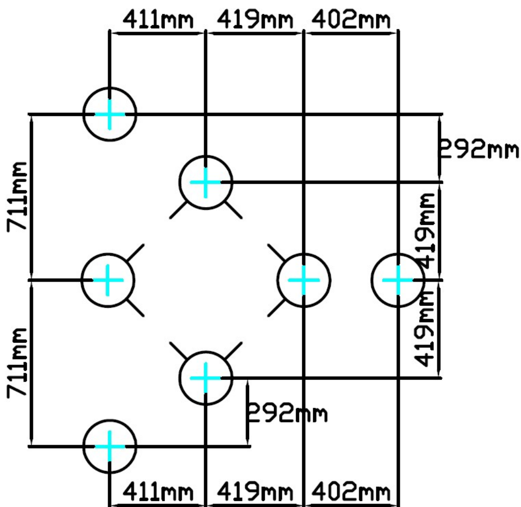
Plattegrond palenplan
