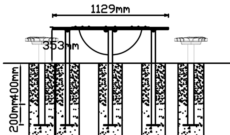
Vooraanzicht
