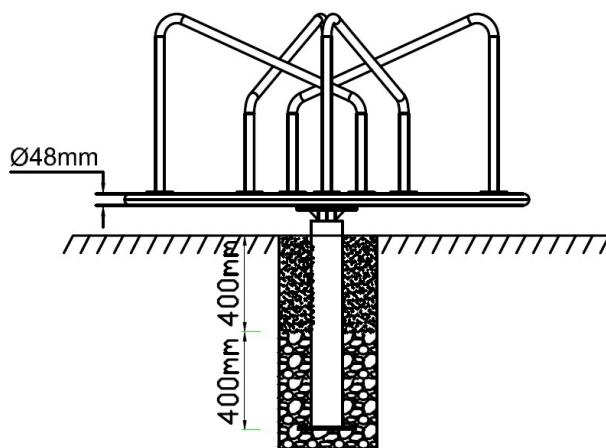
Vooraanzicht
