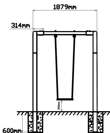
Vooraanzicht
