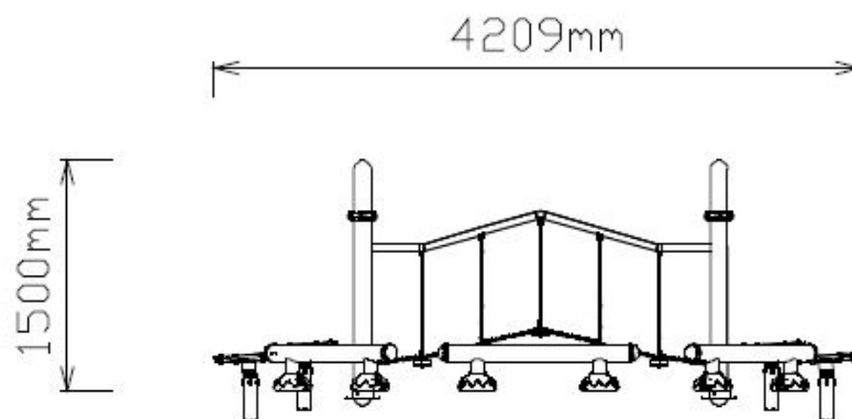
Vooraanzicht
