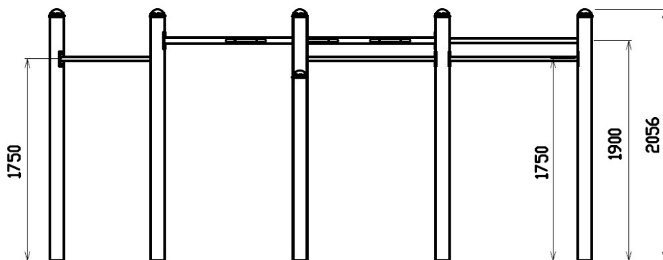
Vooraanzicht
