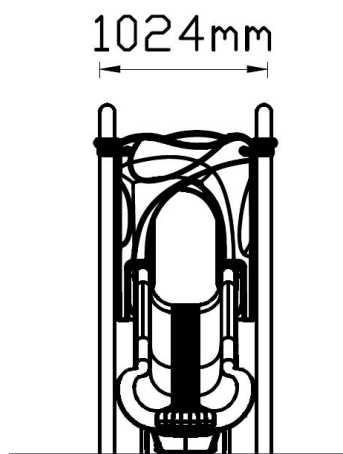
Vooraanzicht
