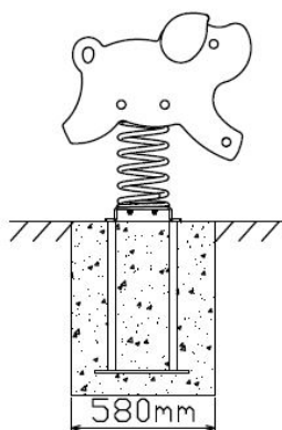
Zijaanzicht
