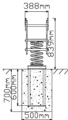
Vooraanzicht
