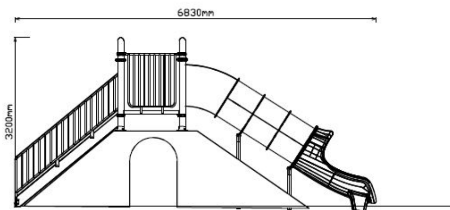
Zijaanzicht
