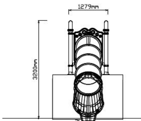
Vooraanzicht
