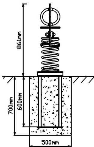
Vooraanzicht
