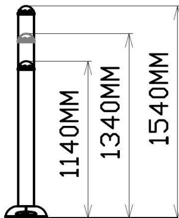
Zijaanzicht
