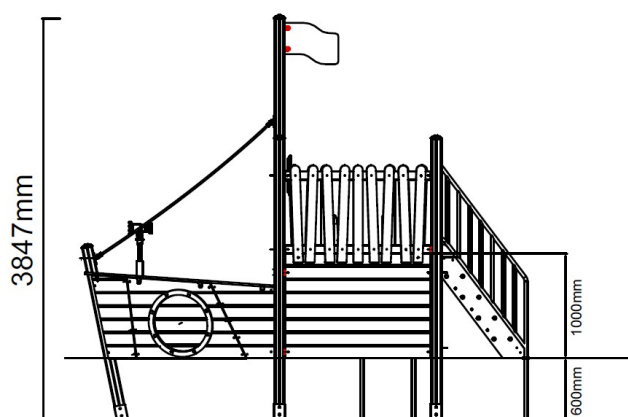
Zijaanzicht
