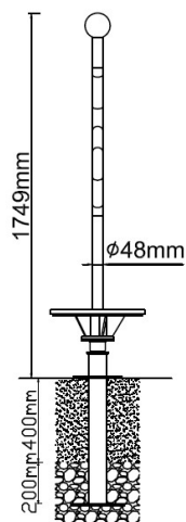
Vooraanzicht
