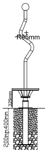
Zijaanzicht
