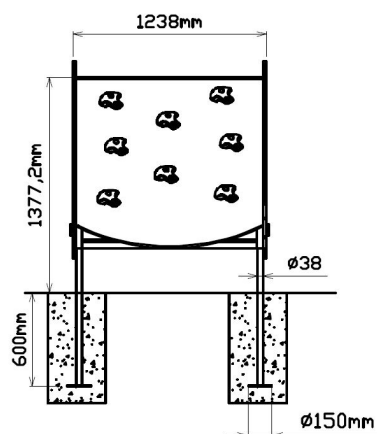
Zijaanzicht
