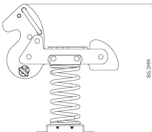
Zijaanzicht
