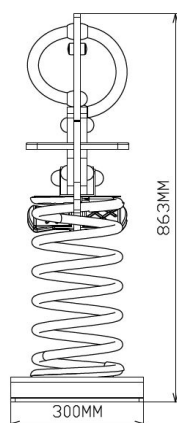
Vooraanzicht
