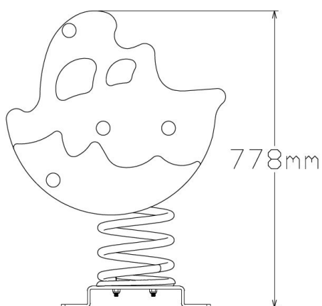
Zijaanzicht
