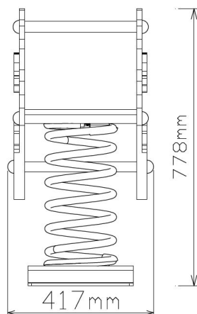
Vooraanzicht
