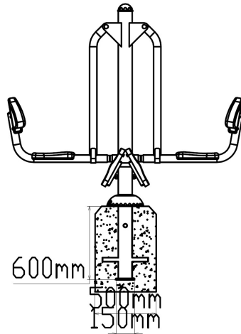
Vooraanzicht
