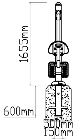
Zijaanzicht
