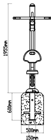
Zijaanzicht
