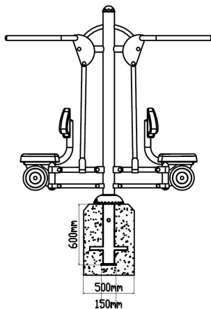
Vooraanzicht
