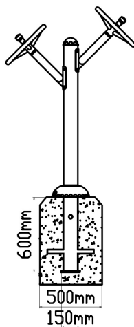
Zijaanzicht
