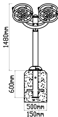
Vooraanzicht
