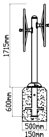
Vooraanzicht
