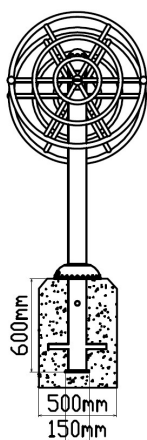
Zijaanzicht
