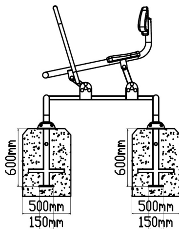
Vooraanzicht
