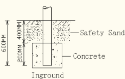
Betonfundatie
