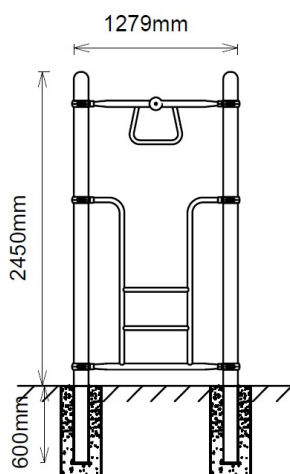
Zijaanzicht
