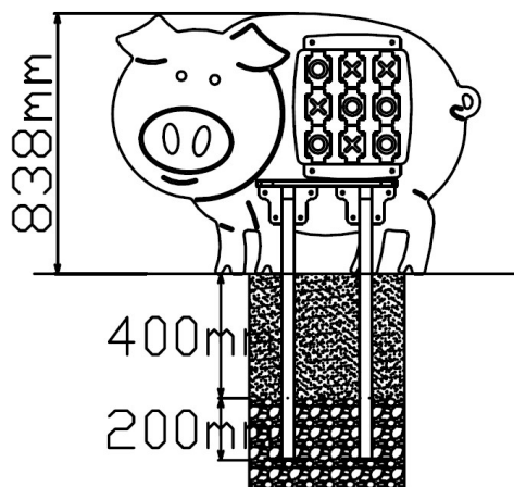
Vooraanzicht
