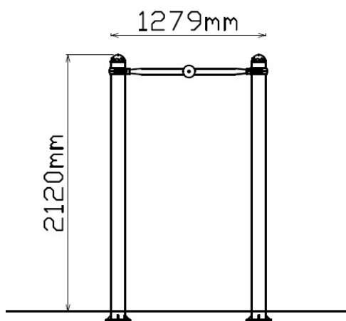
Zijaanzicht
