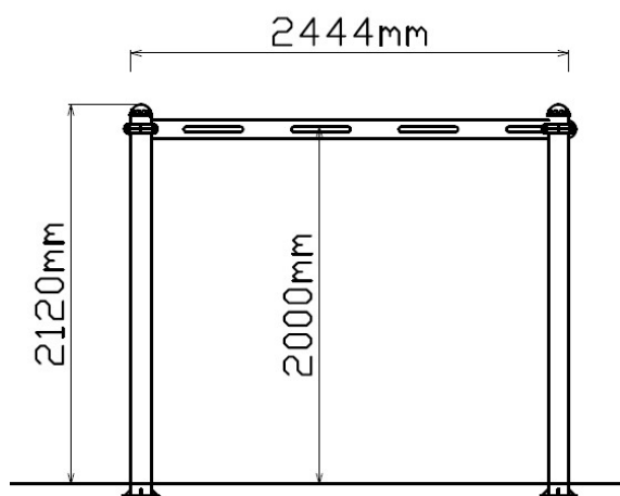
Vooraanzicht
