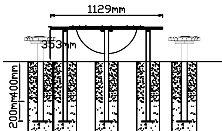
Vooraanzicht
