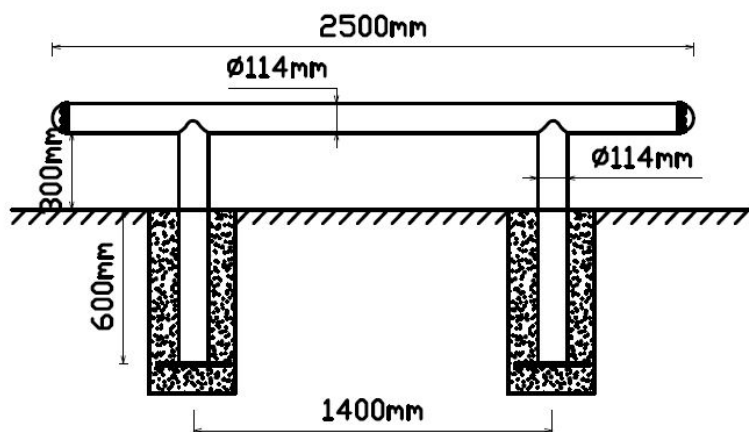
Vooraanzicht
