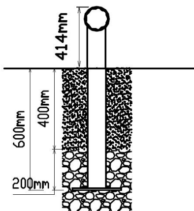
Zijaanzicht
