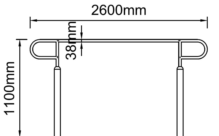
Vooraanzicht
