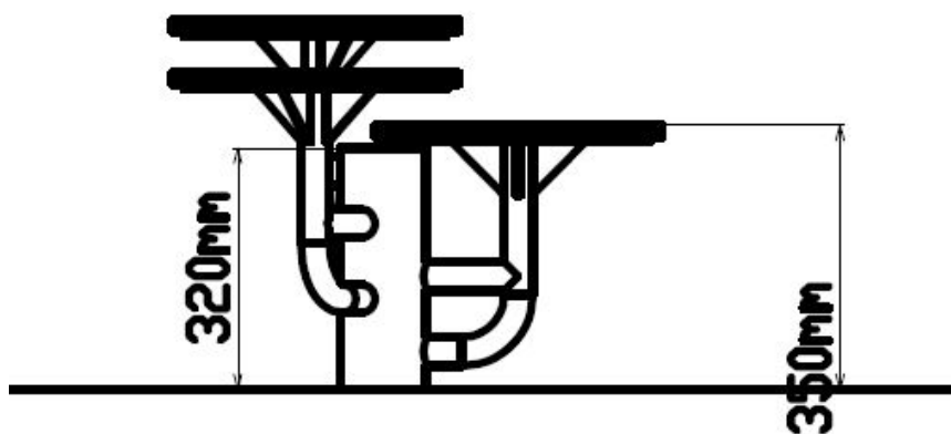
Vooraanzicht
