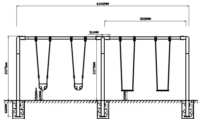
Vooraanzicht
