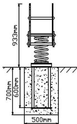
Vooraanzicht
