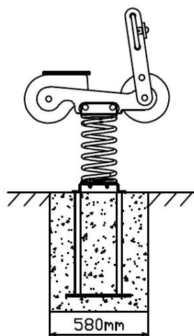
Zijaanzicht
