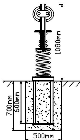
Vooraanzicht
