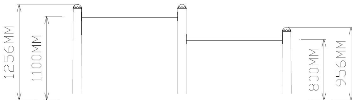
Vooraanzicht
